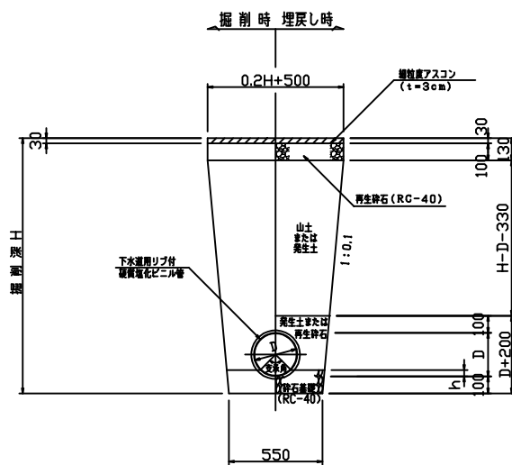
掘削深 H \leq 1.5\text{m} (素掘り部)
