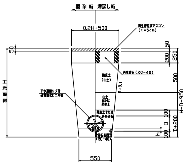
掘削深 H \leq 1.5\text{m} (素掘り部)
