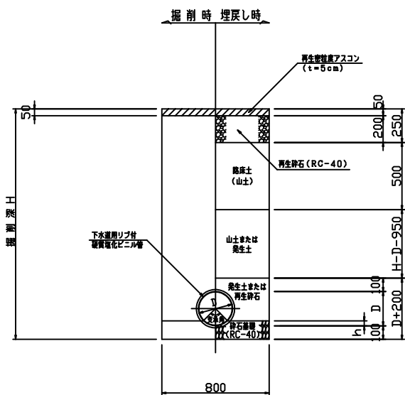
掘削深 H > 1.5\text{m} (矢板部)
