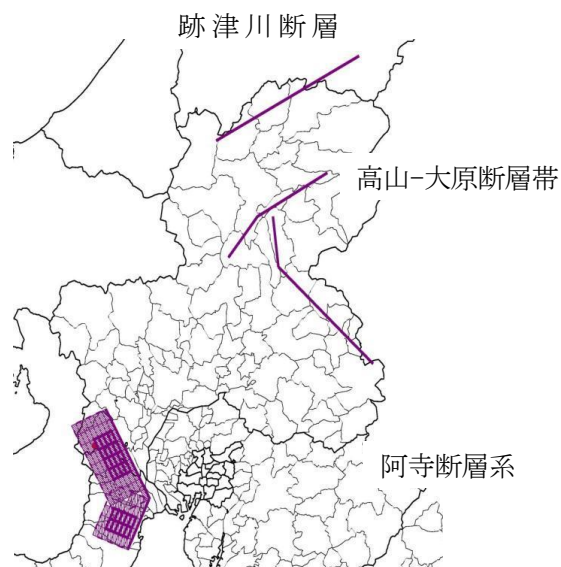
内陸直下型地震断層位置図
