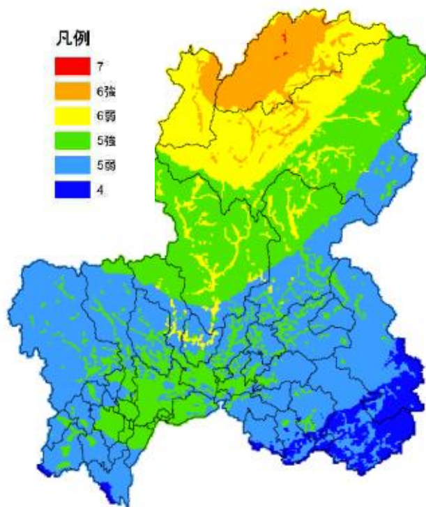
震度分布図
