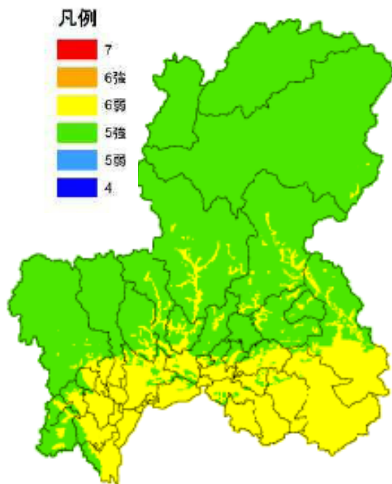
震度分布図
