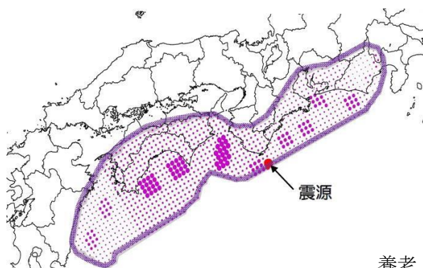
南海トラフ巨大地震(海溝型地震)断層位置図
