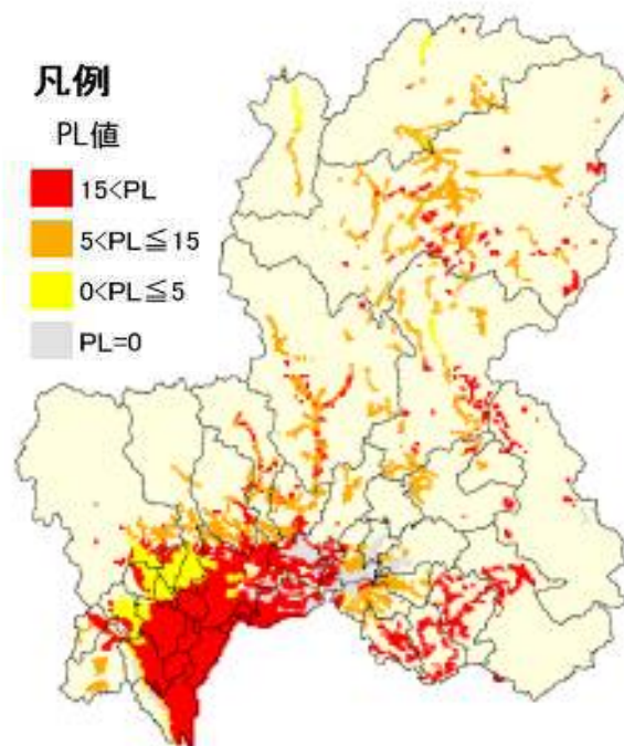
液状化分布図
