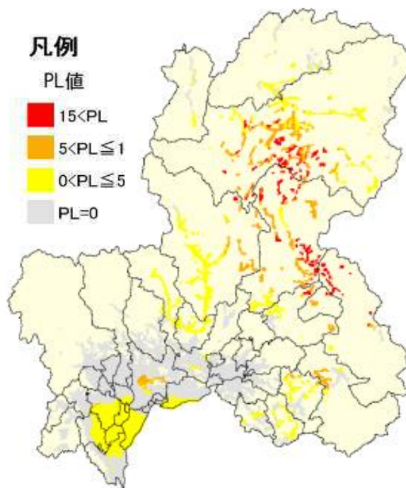
液状化分布図
