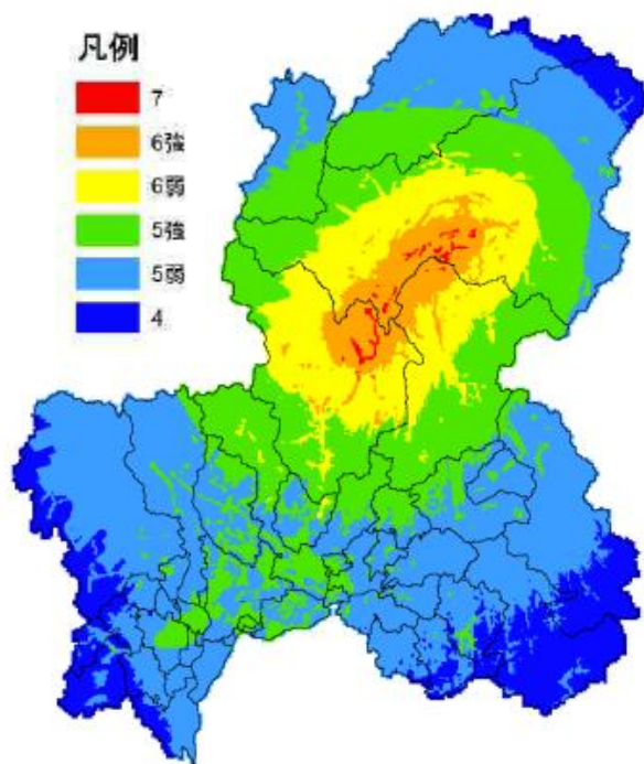
震度分布図
